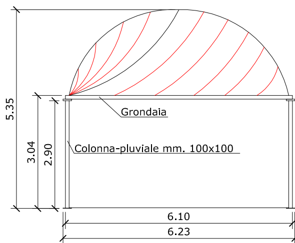
- PROSPETTO
