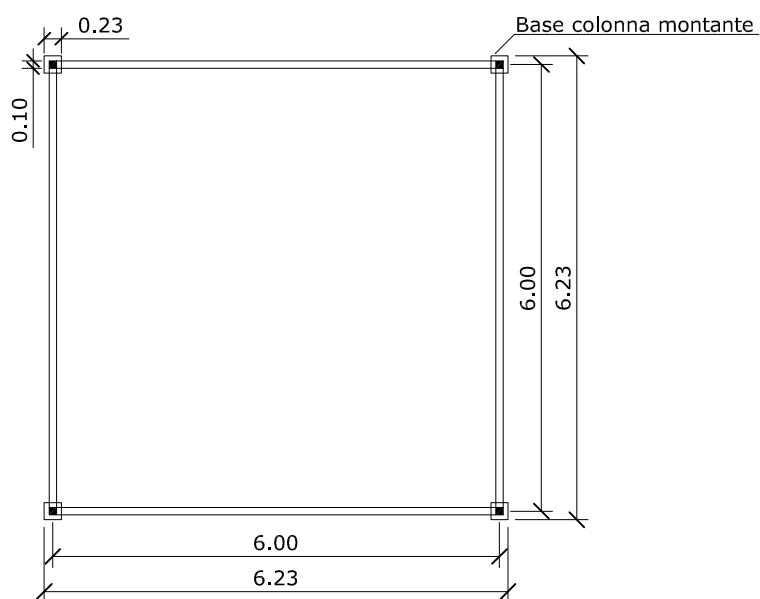
- PIANTA
